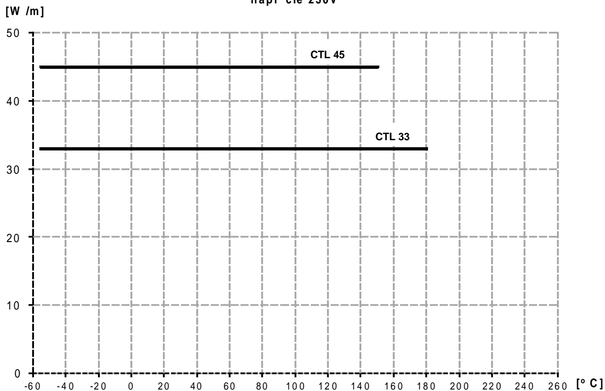
Charakterystyka mocy grzewczej napięcie 230V
